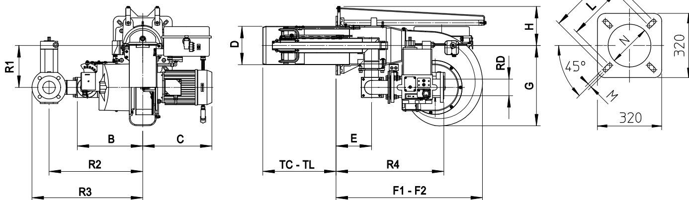
РАЗМЕРЫ [мм]
